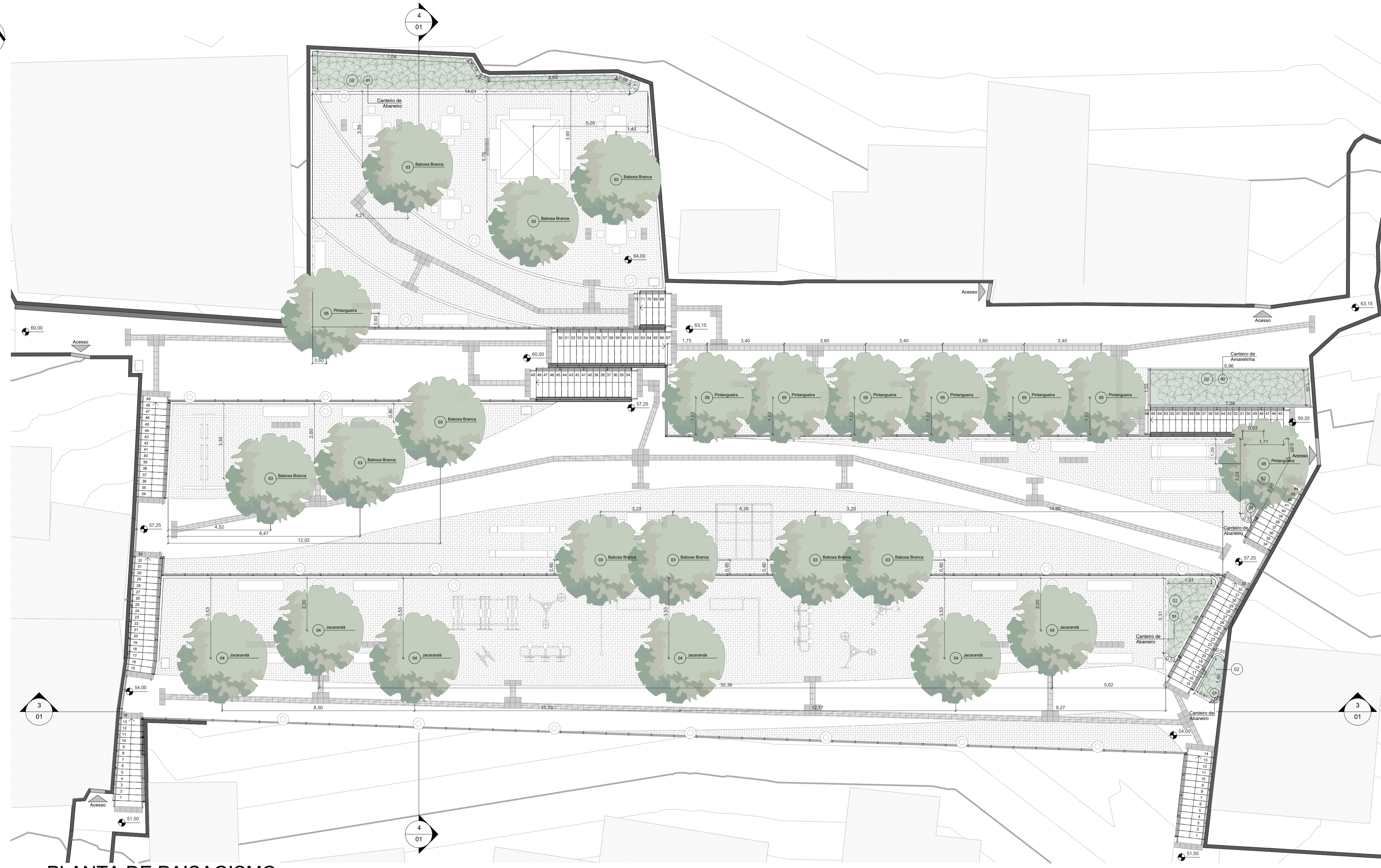
1 PLANTA DE PAISAGISMO 1 : 100
