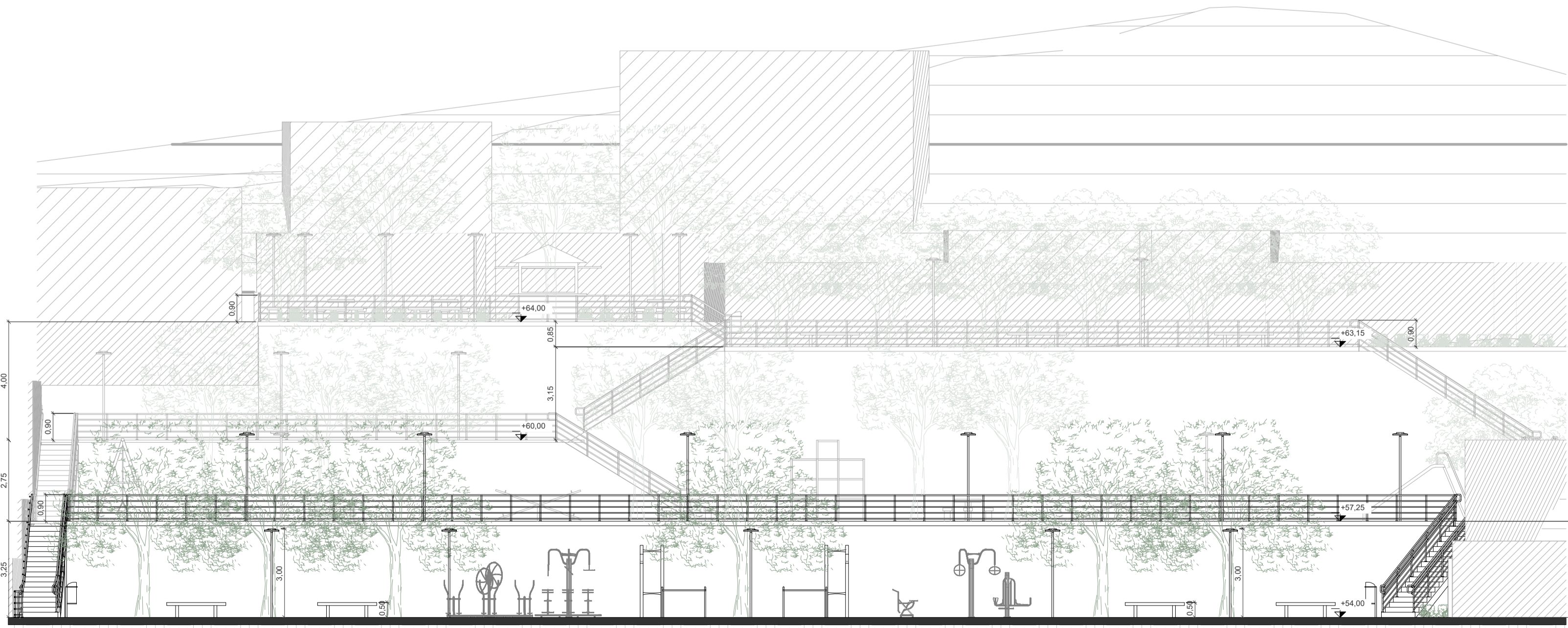
3 CORTE LONGITUDINAL 1 : 125
