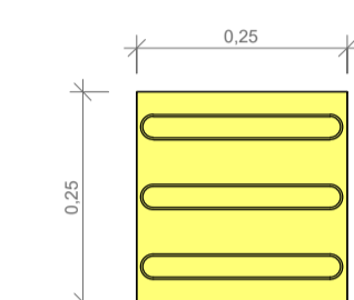
2 DET - SINALIZAÇÃO PODOTÁTIL 1 : 10
