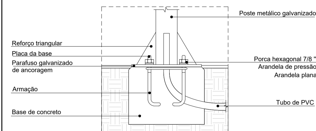
2 DET - FIXAÇÃO DE POSTE PEDONAL 1 : 25
