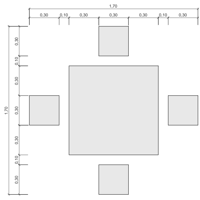
4 DET - MESA COM 4 BANCOS 1 : 20
