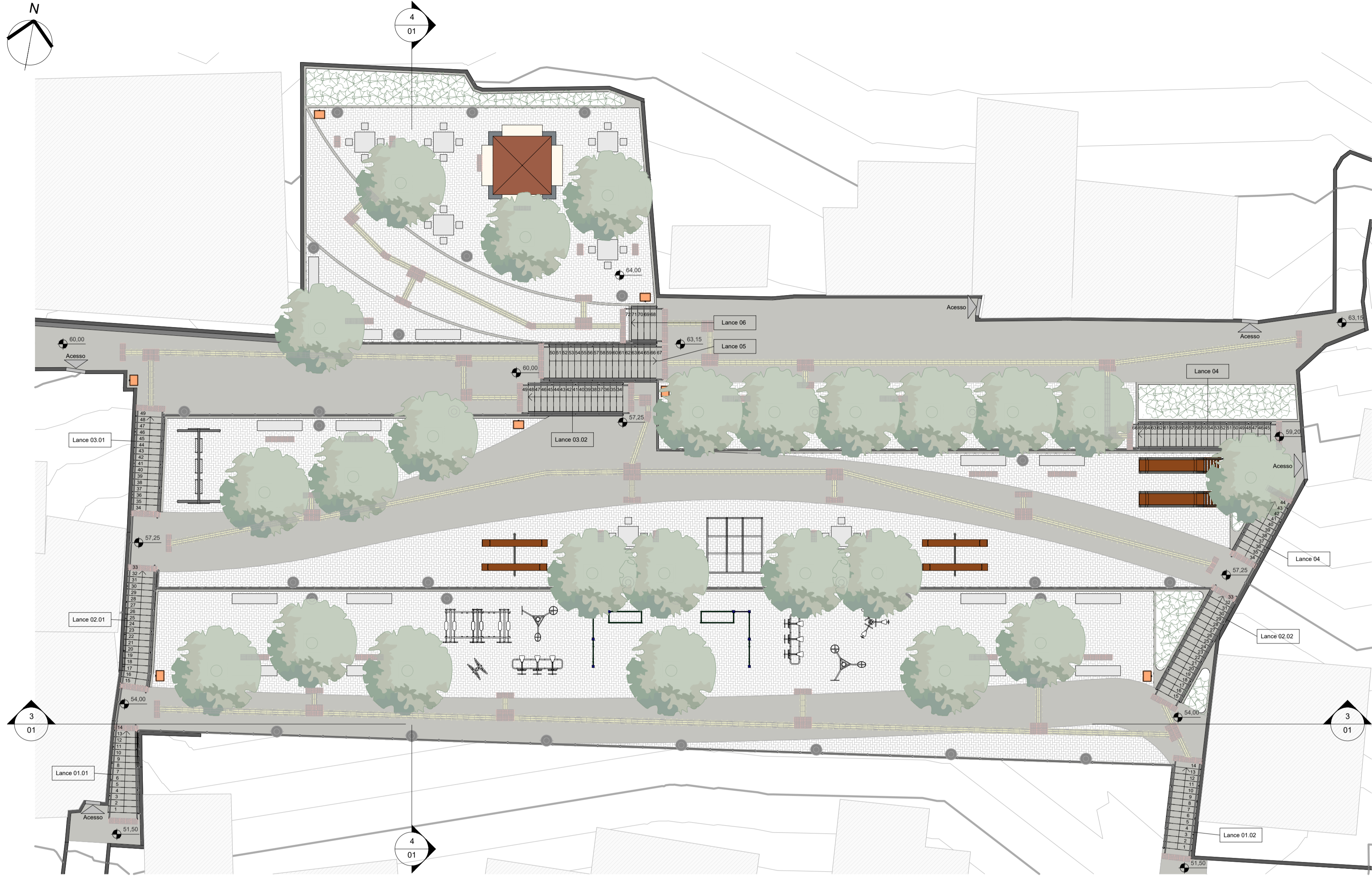
1 PLANTA DE SITUAÇÃO 1 : 125
