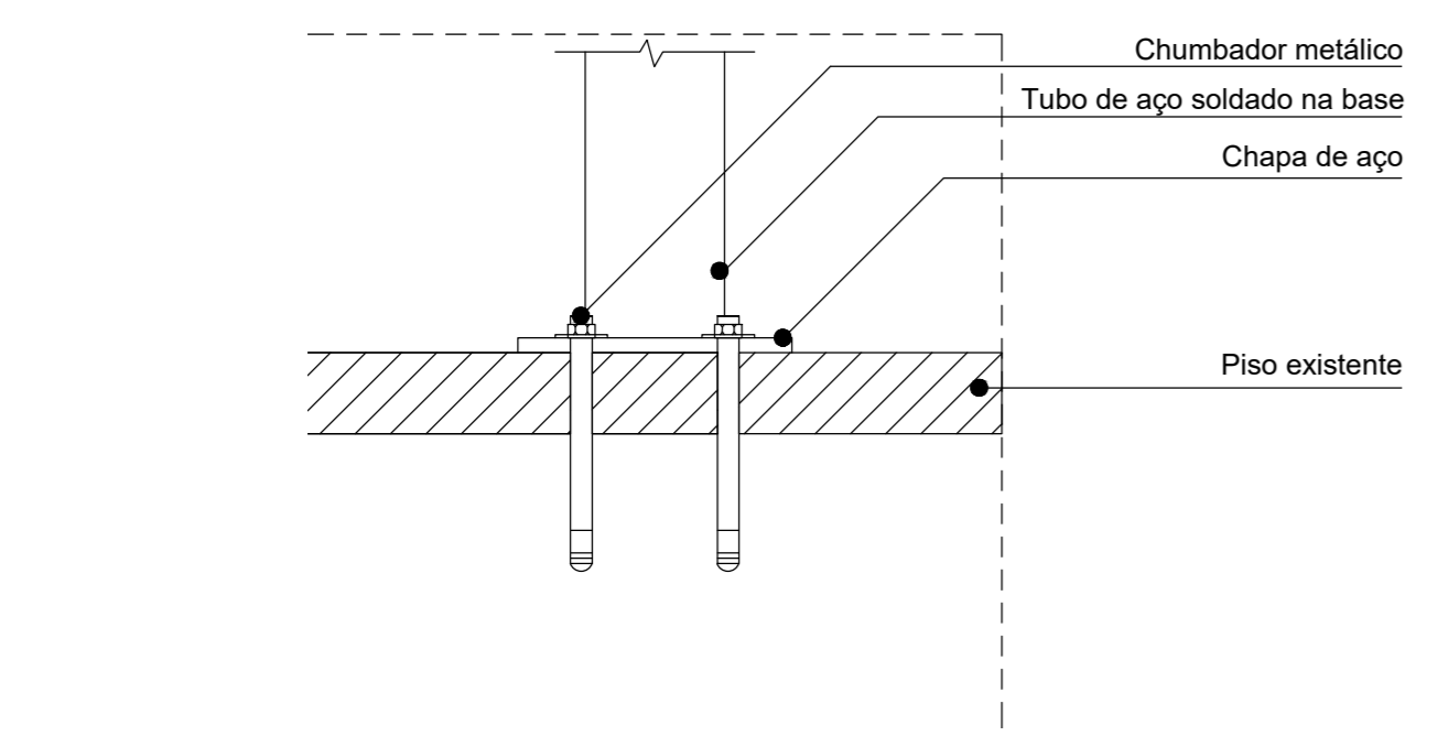
2 DET. FIXAÇÃO GUARDA CORPO PISO 1 : 3
