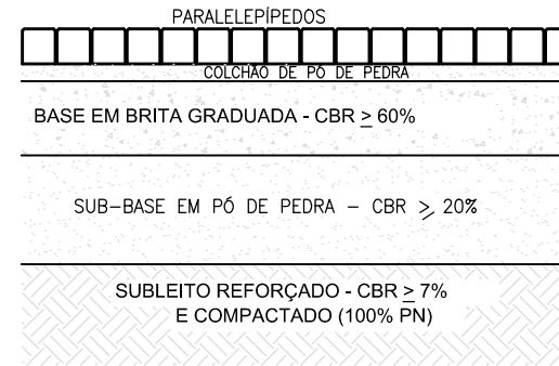
ESQUEMA DO PAVIMENTO INTERTRAVADO
