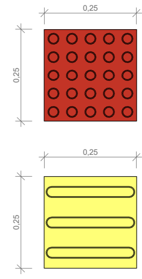
1 DETALHE DE SINALIZAÇÃO PODOTÁTIL ESCALA 1:10
