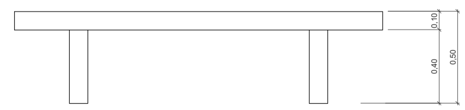
2 DETALHAMENTO - BANCO DE CONCRETO 1 : 20
