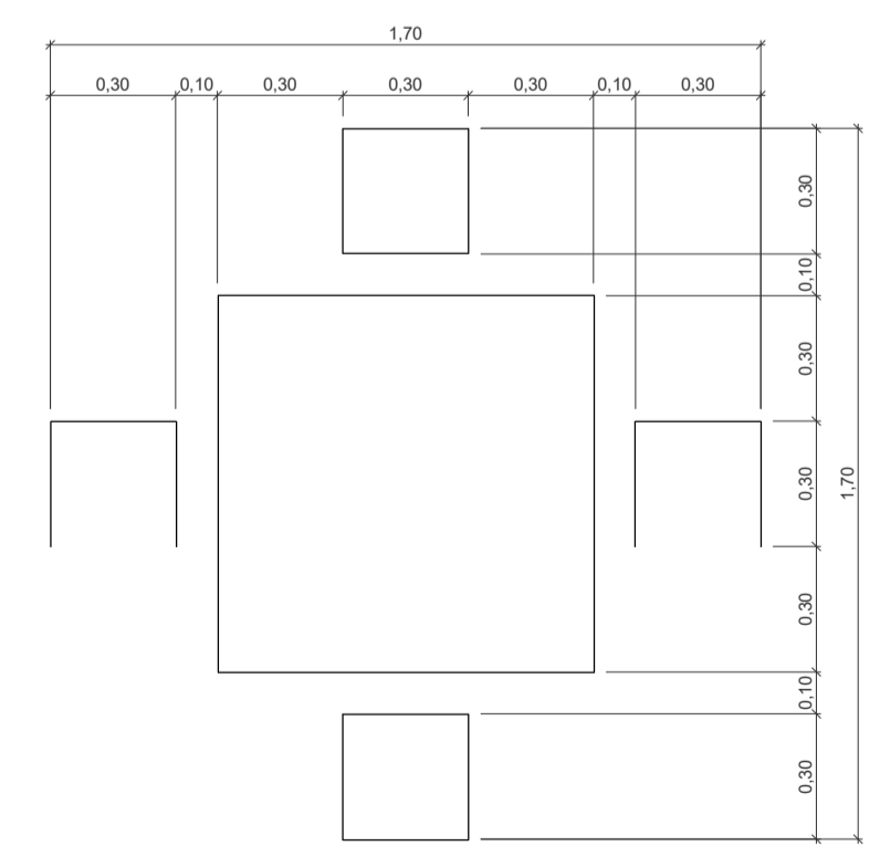
3 DETALHAMENTO - MESA COM BANCOS 1 : 20
