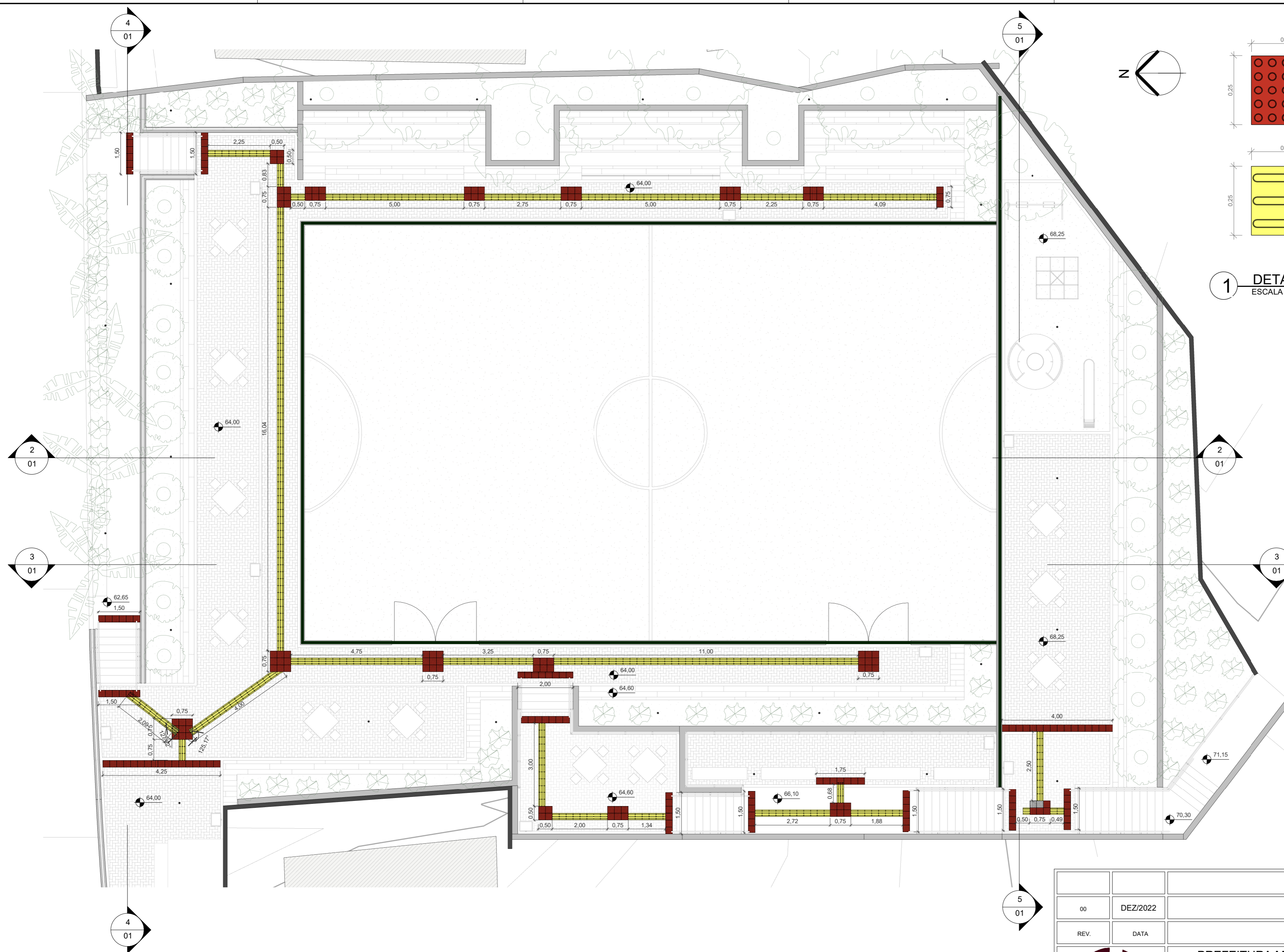
1 PLANTA DE ACESSIBILIDADE 1:100
