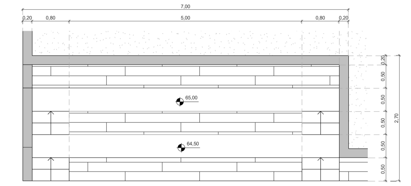
4 DETALHAMENTO - ARQUIBANCADA 1 : 50
