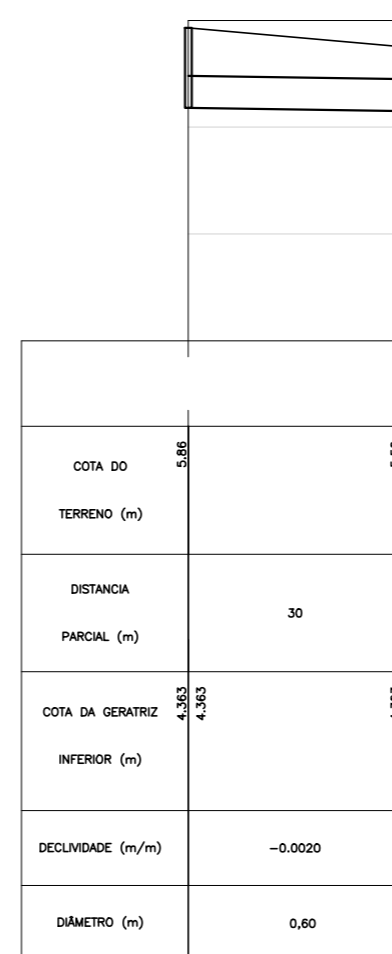
TRECHO PV23 - PV19 ESCALA VERTICAL: 1:100 ESCALA HORIZONTAL: 1:1000
