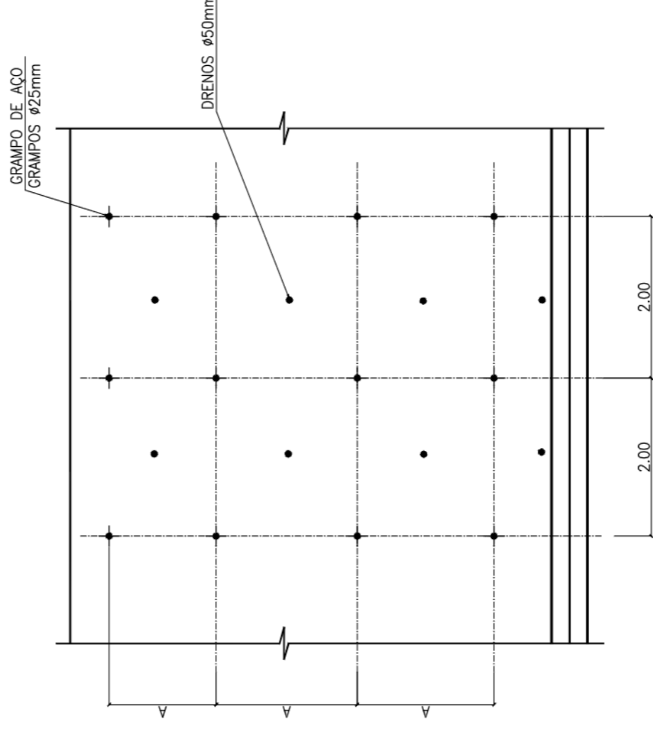
02 DETALHE DE SOLO GRAMPEADO ESC: 1/50
