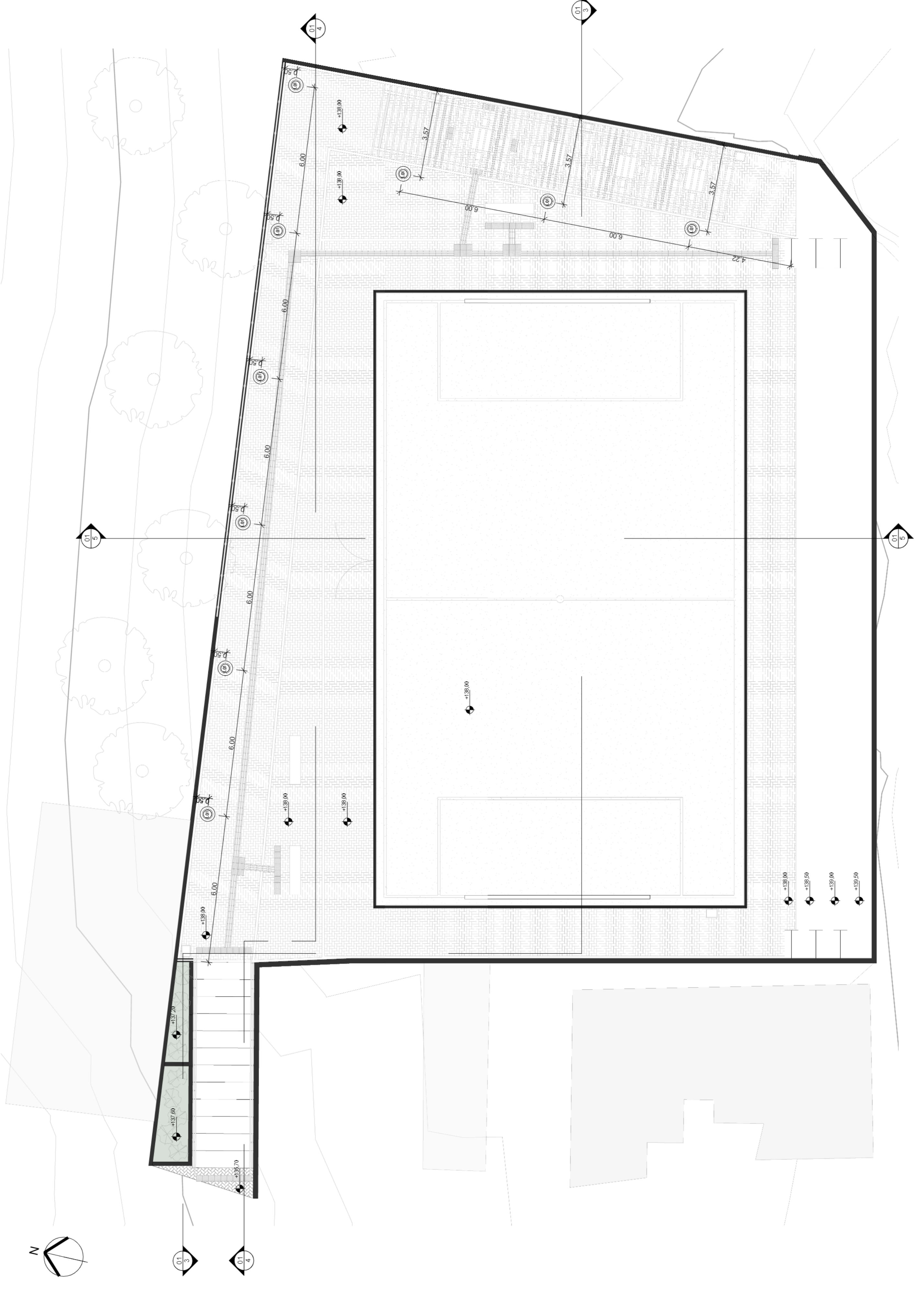
1 PLANTA DE ILUMINAÇÃO 1 : 100
