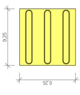
2 DET. - SINALIZAÇÃO PODOTÁTIL 1 : 10
