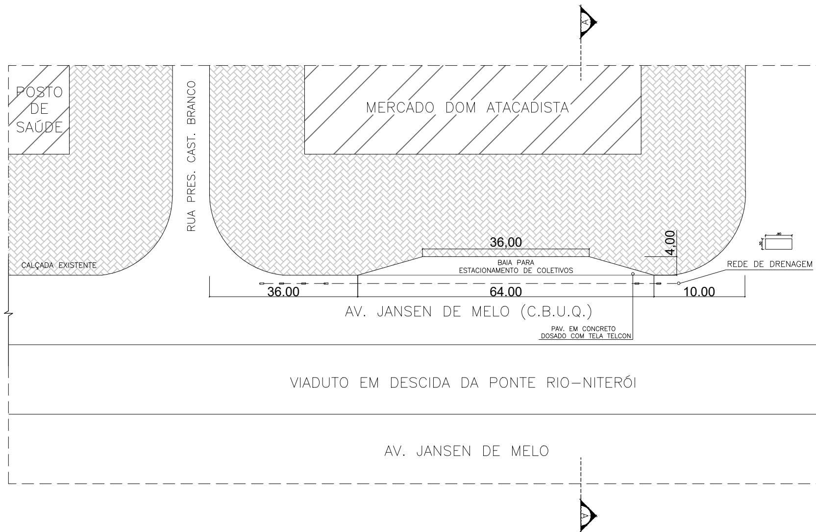
1 PLANTA BAIXA ESQUEMÁTICA ESC: 1/800
