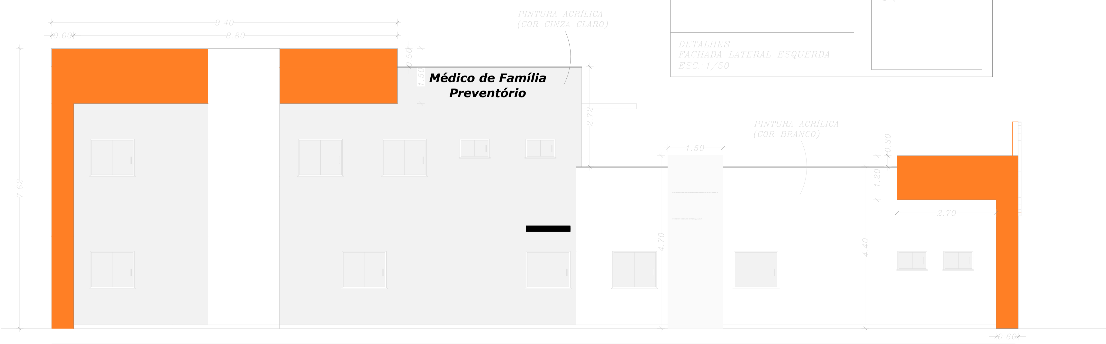
FACHADA LATERAL ESQUERDA ESC.: 1/50
