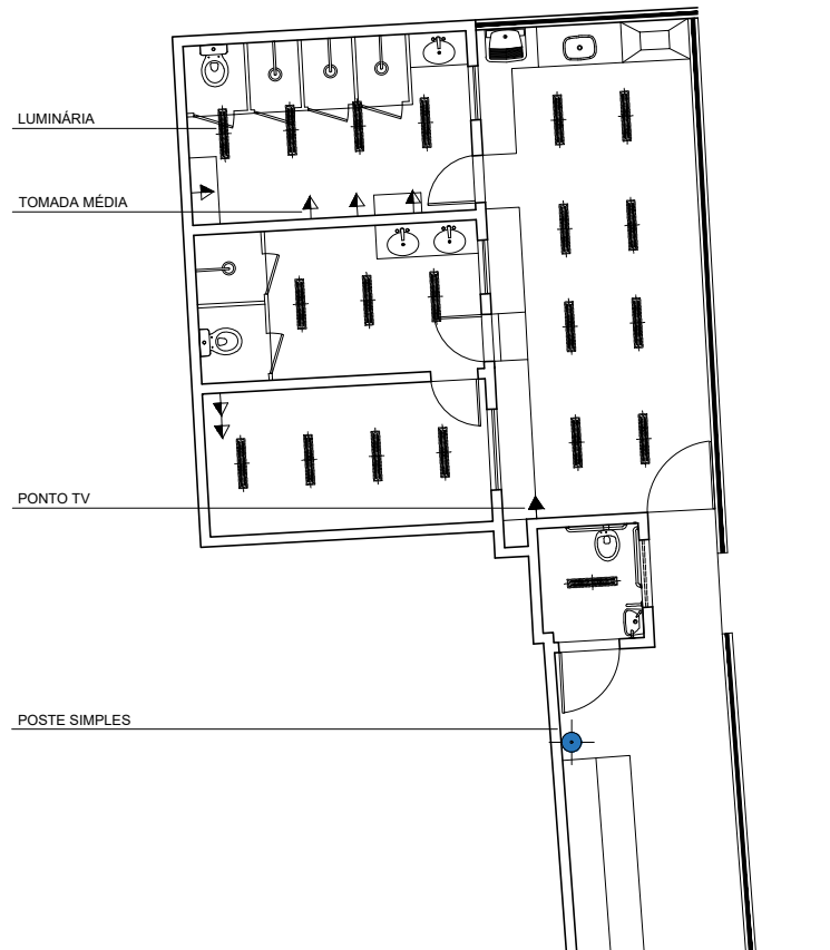
01 PLANTA BAIXA - LOCAÇÃO DE PONTOS ESCALA 1:125
