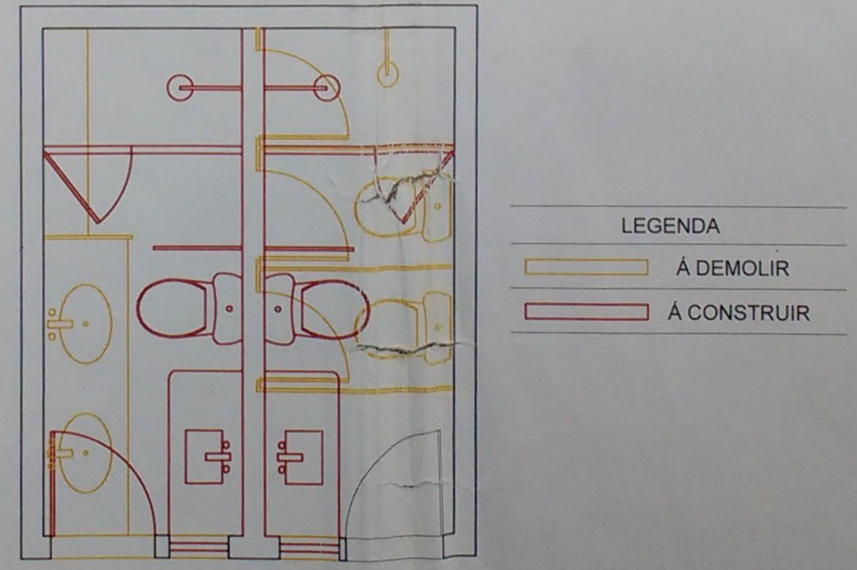
4 PLANTA BAIXA DEMOLIR/CONSTRUIR
