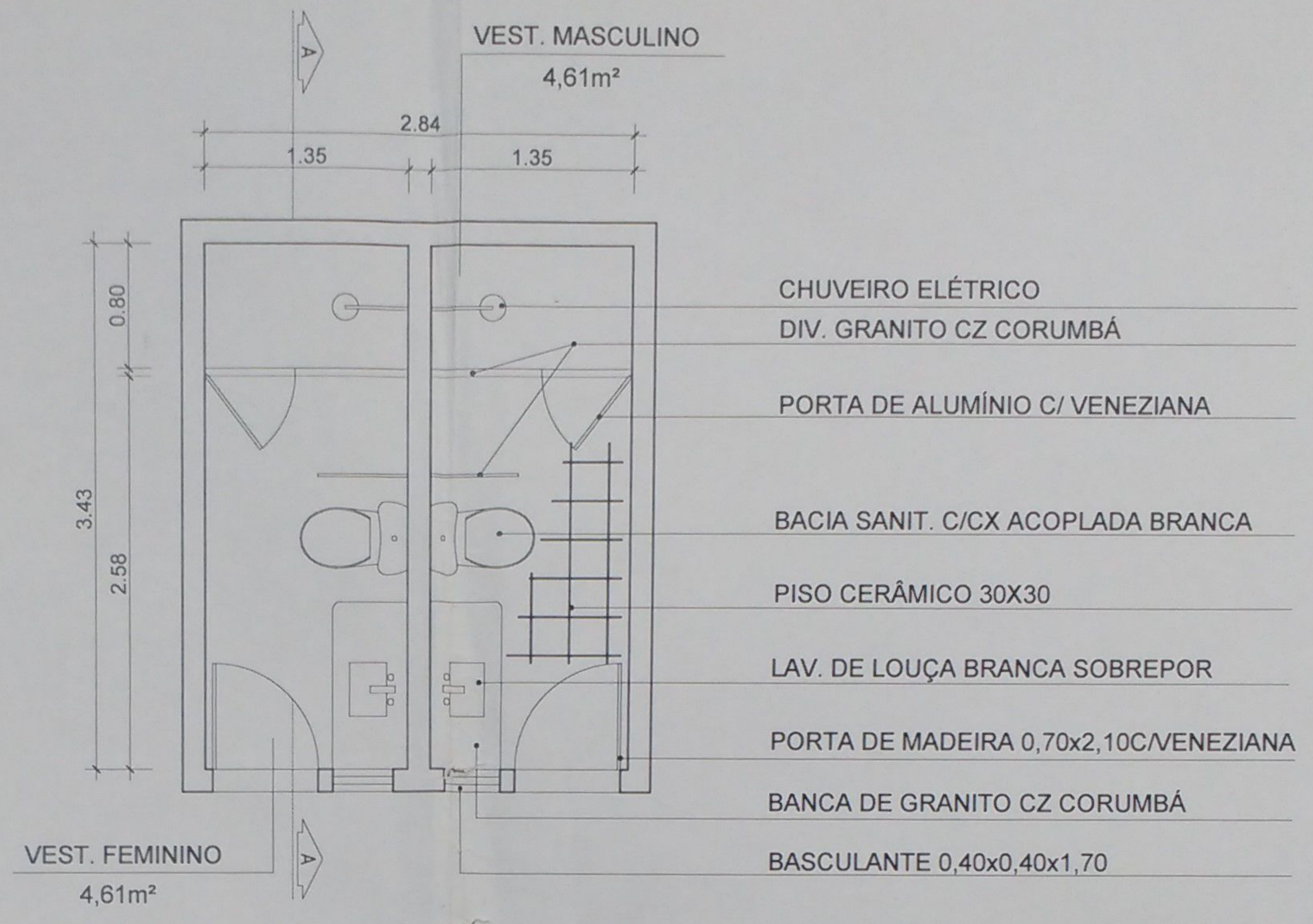
2 PLANTA BAIXA - VESTIÁRIO REFORMA
