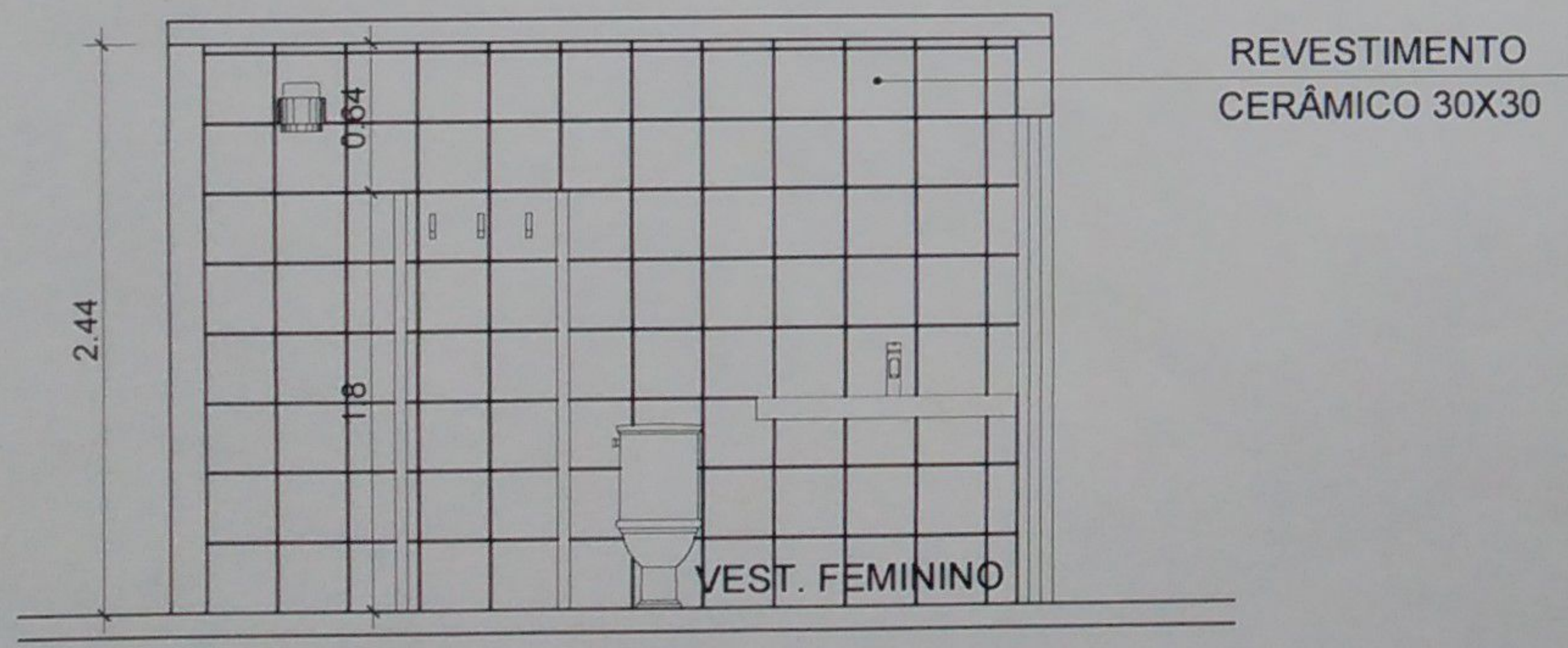
3 CORTE AA
