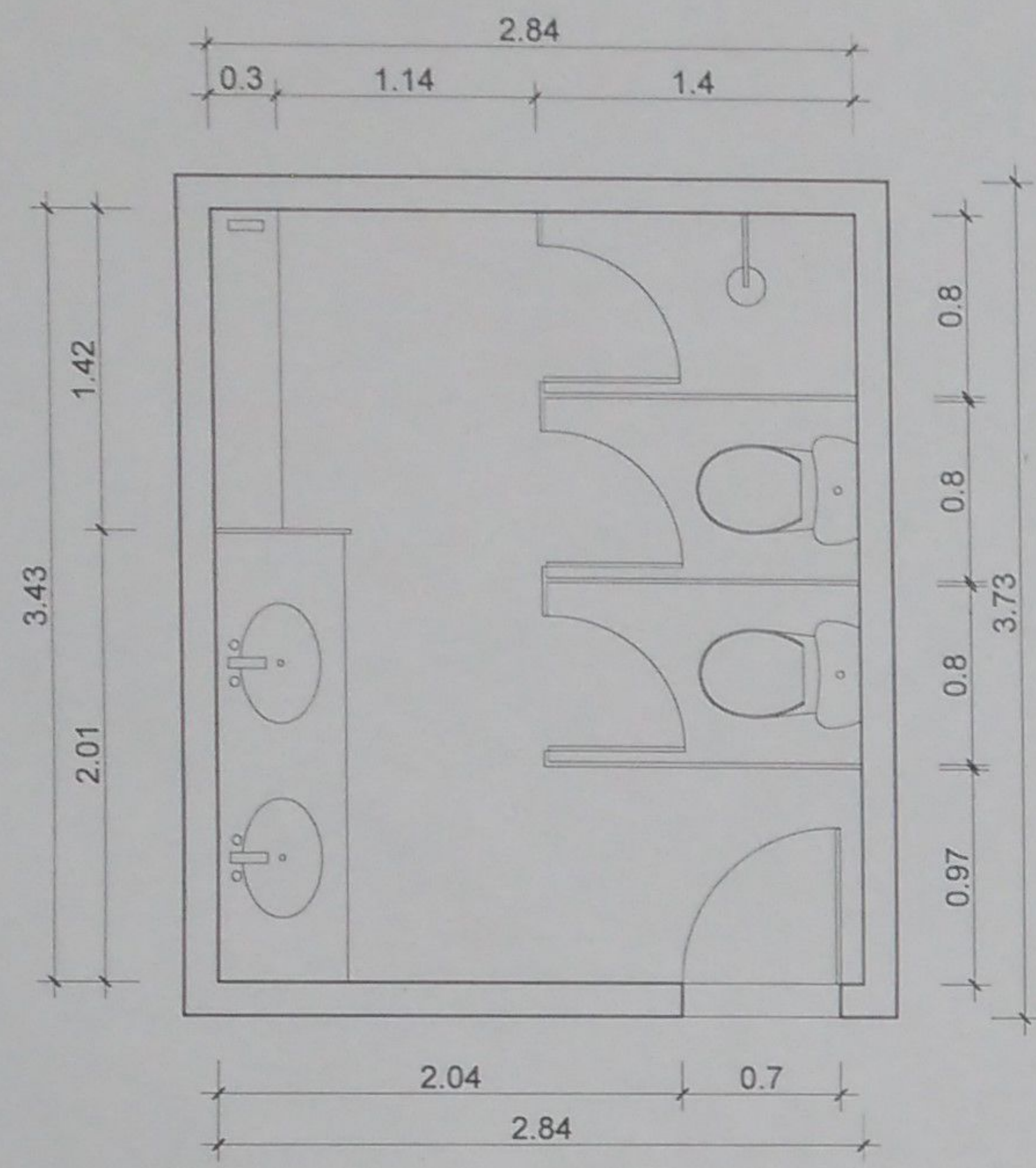
1 PLANTA BAIXA - VESTIÁRIO ATUAL
