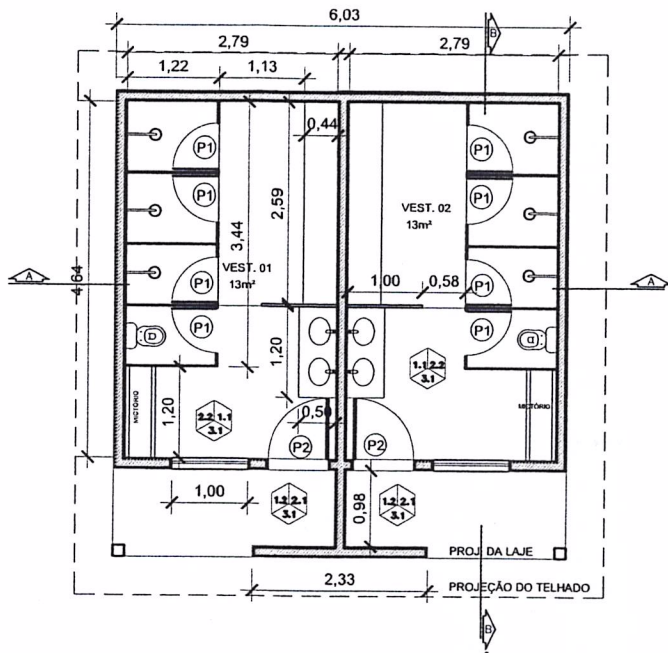
01 PLANTA BAIXA VESTIÁRIO ESC.: 1/100
