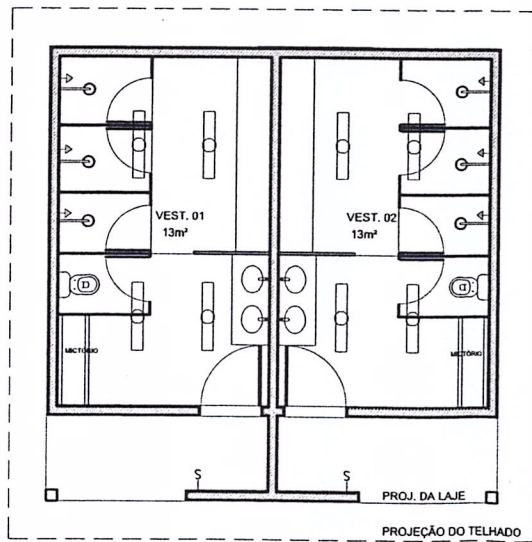
05 LOCAÇÃO DOS PONTOS DE ELÉTRICA ESC.: 1/100
