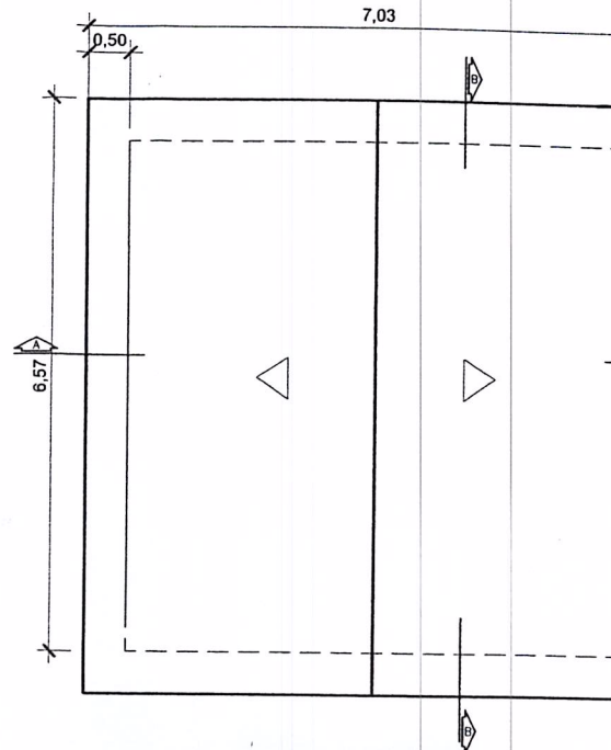
02 PLANTA DE COBERTURA ESC.: 1/100
